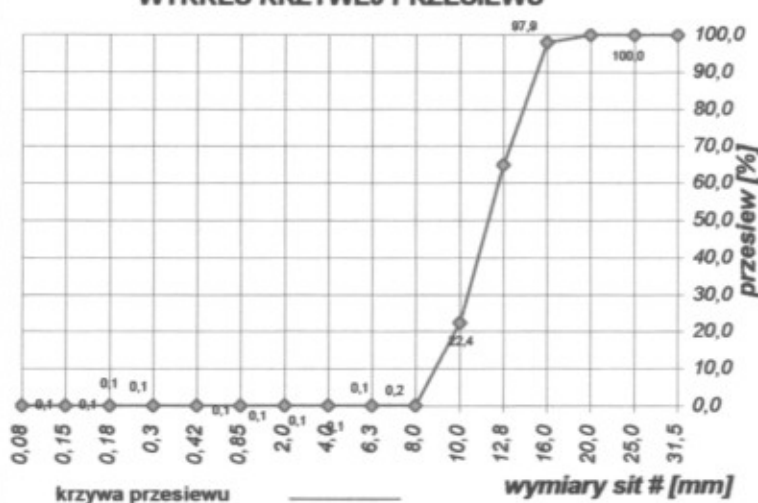
WYKRES KRZYWEJ PRZESIEWU
