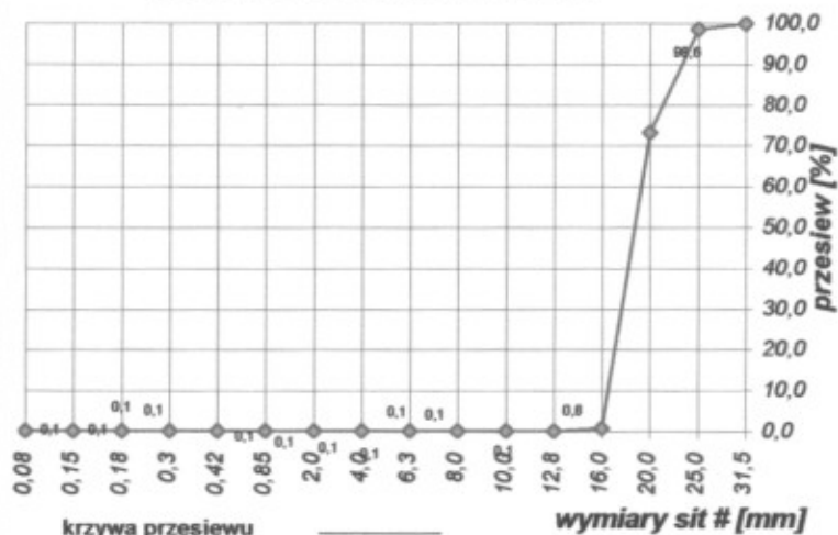
WYKRES KRZYWEJ PRZESIEWU
